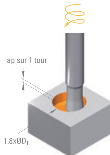
Calcul des valeurs d'hélice: ap \text{ sur 1 tour} = \pi \times D_1 \times \tan \alpha
